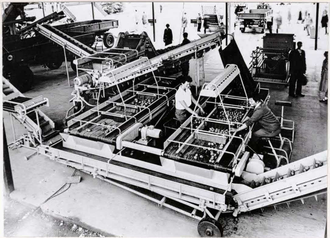
Kartoffelsortierer K 710
