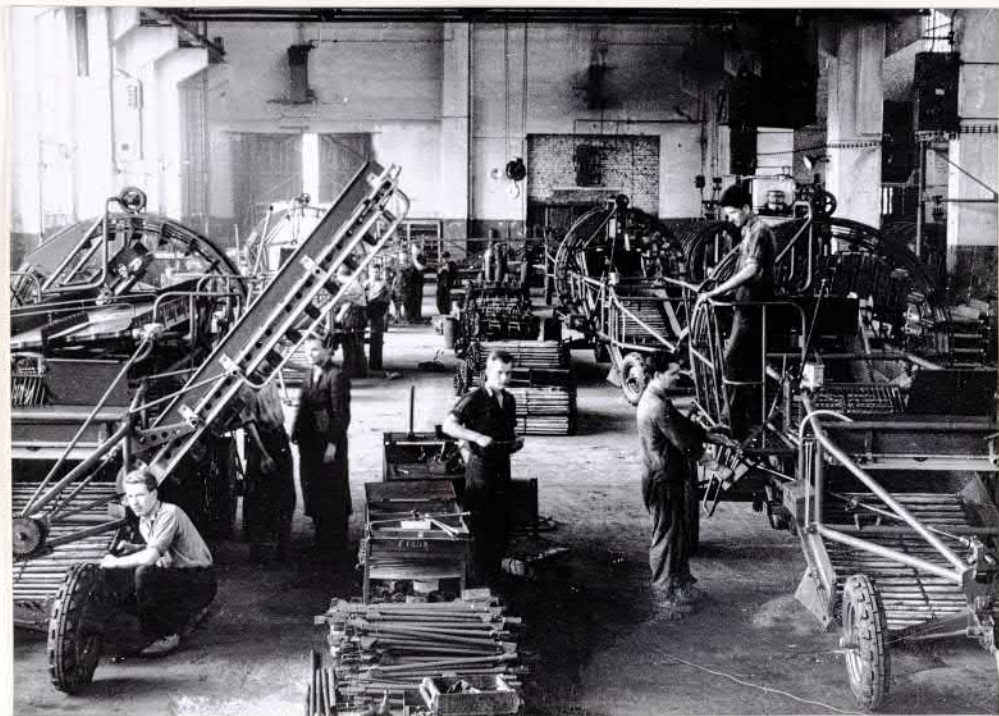
Taktstraße der Endmontage Kartoffelvollertemaschine E 675
