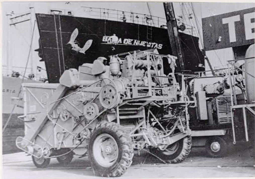
Ausschiffung des Mähreschers E 177 im Hafen von Havanna
