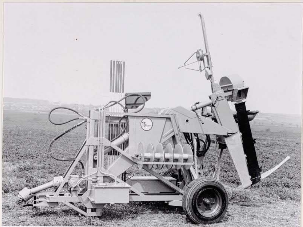
Maulwurfdränmaschine B 750
