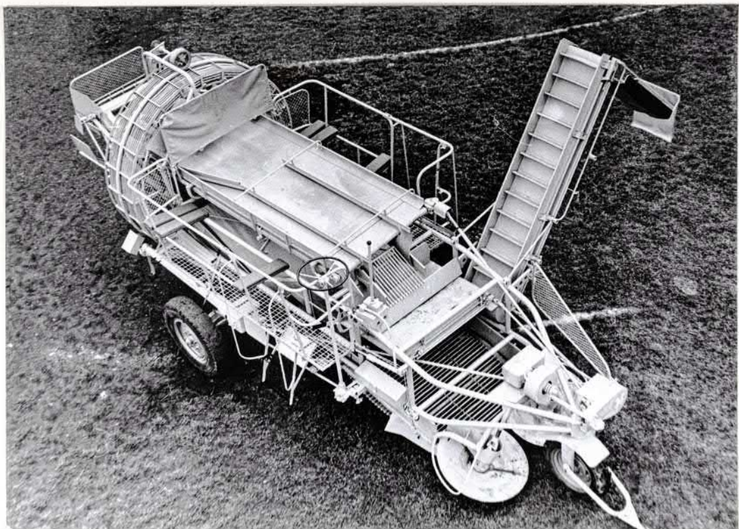
Kartoffelvollerntemaschine E 675/1
