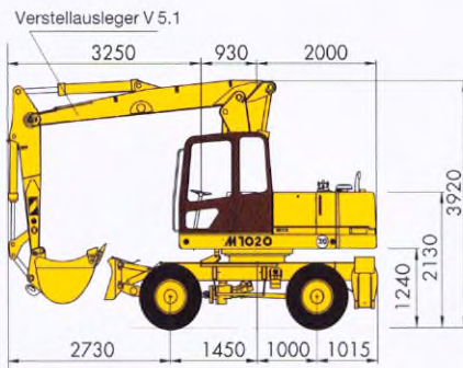
Transportmaße
